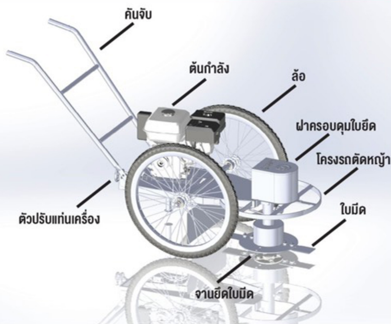
ภาพประกอบชิ้นส่วน รถตัดหญ้า
